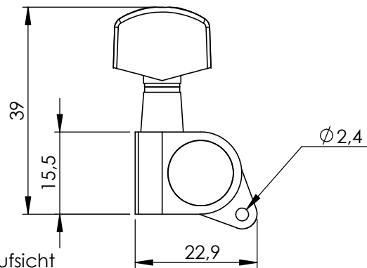
Vorderansicht front view
