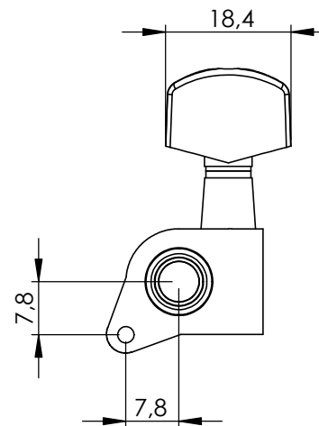
Unteransicht bottom view
